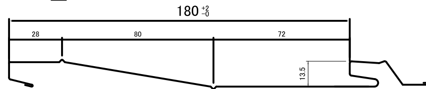
横葺 180 M型
