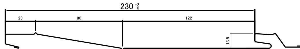
横葺 230 M型
