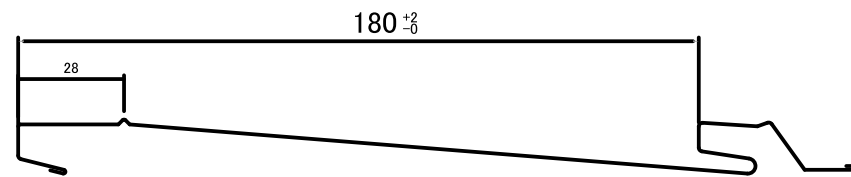
横葺 180 フラット型
